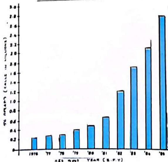
ባለፉት ስድስት ዓመታት ውስጥ የልማት ፕሮግራም ስልጣን SIXTH DEVELOPMENT PROGRAMME - INTERNATIONAL TELEPHONE TRAFFIC (OUT GOING)
